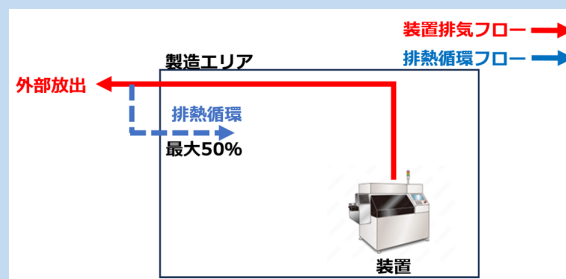
(排熱利用フロー図)
